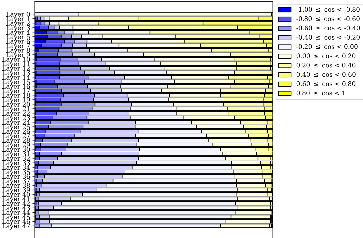
gpt2-xl
