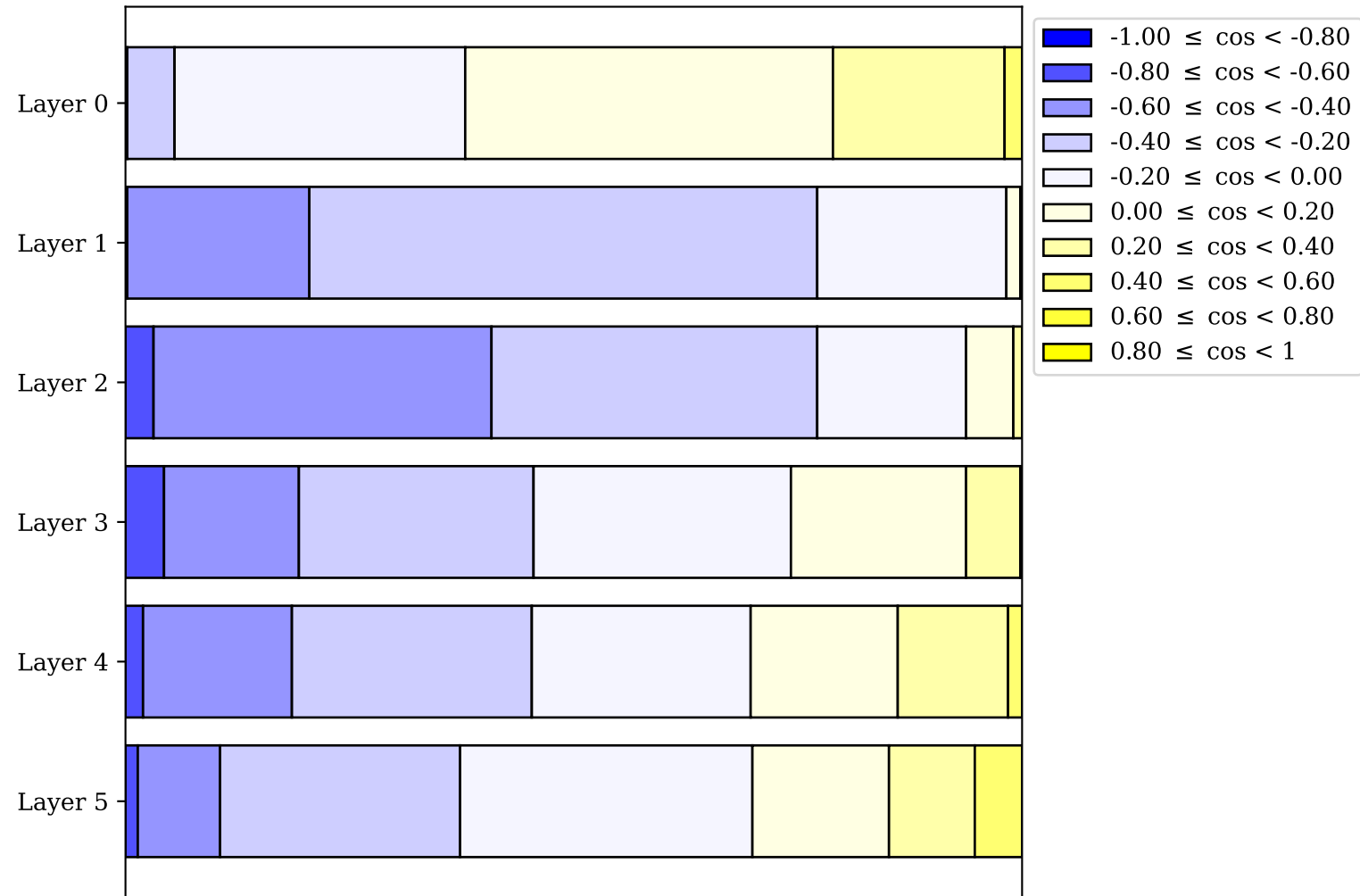
pythia-14m
