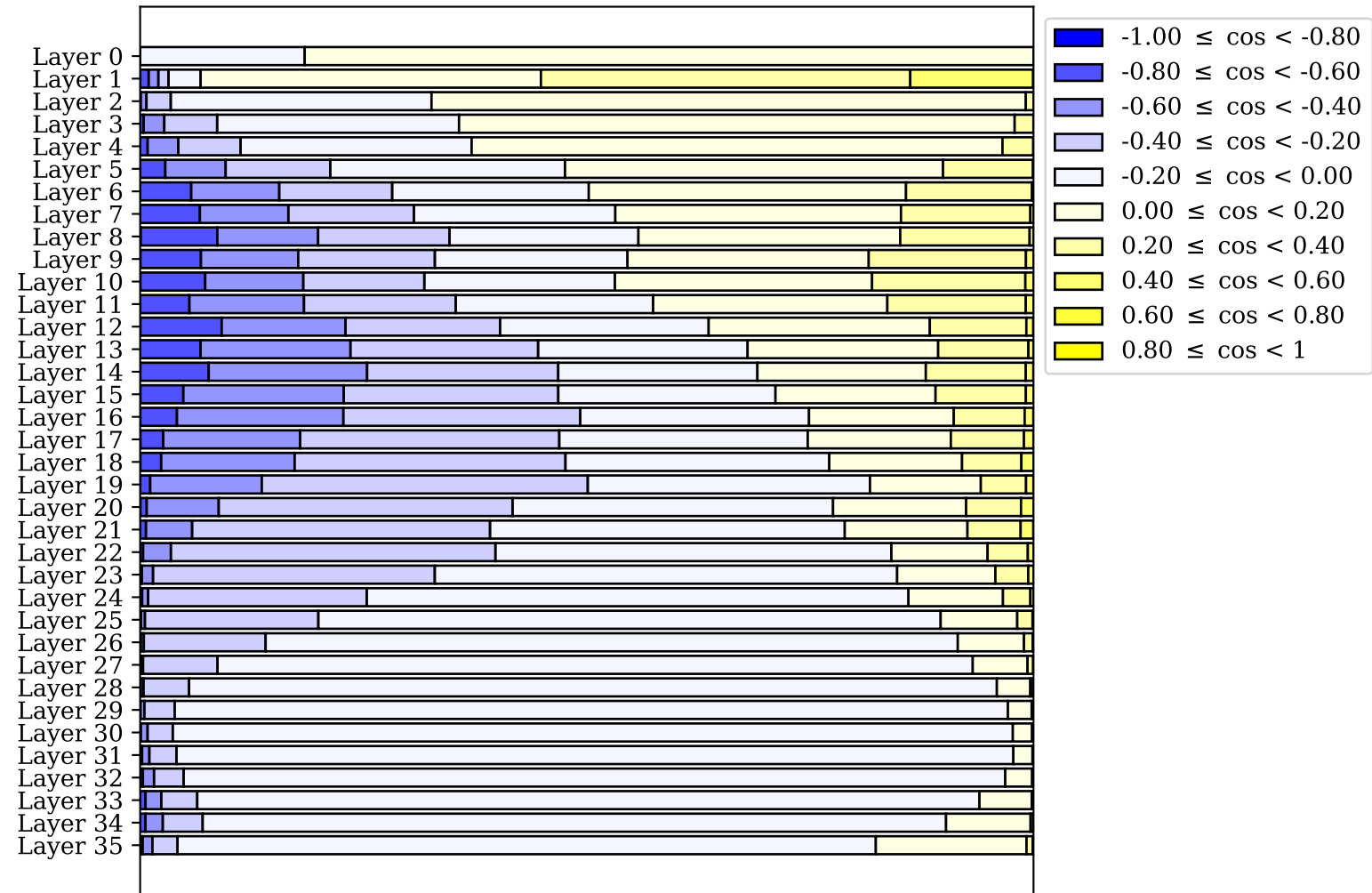
pythia-12b
