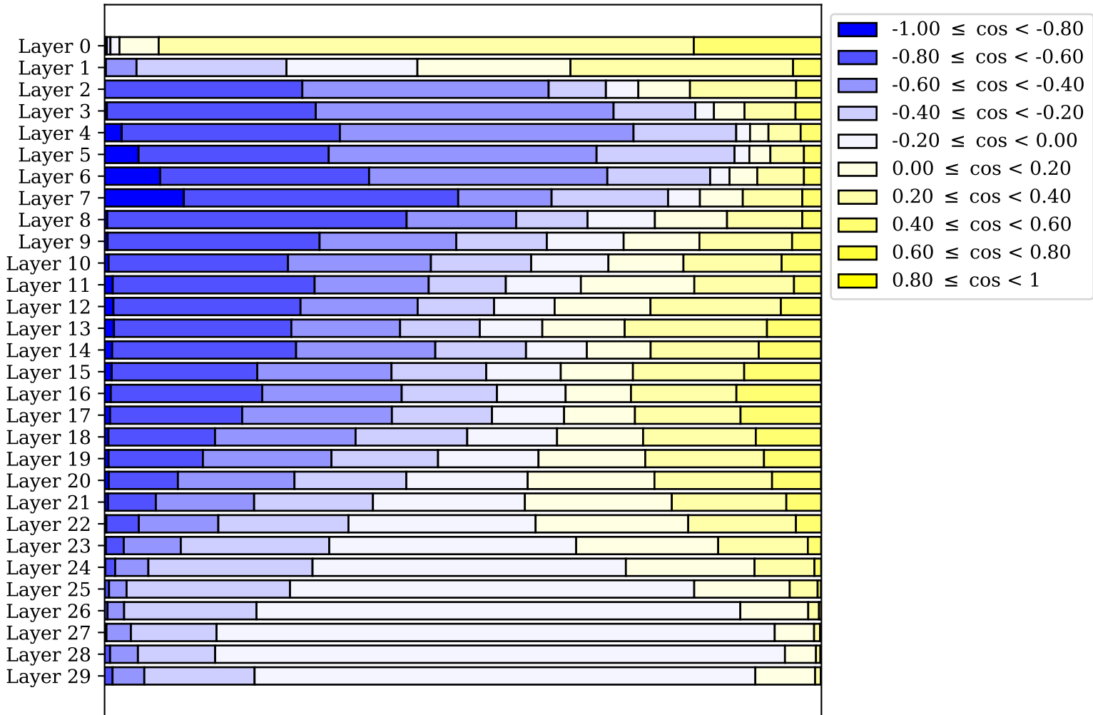
bloom-7b1
