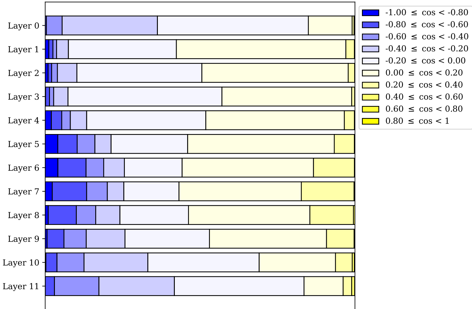
opt-125m
