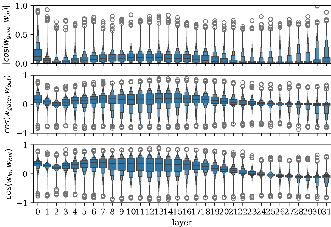
Llama-2-7b
