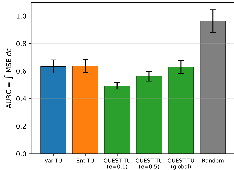
t3 ( n_{seeds}=10 )
