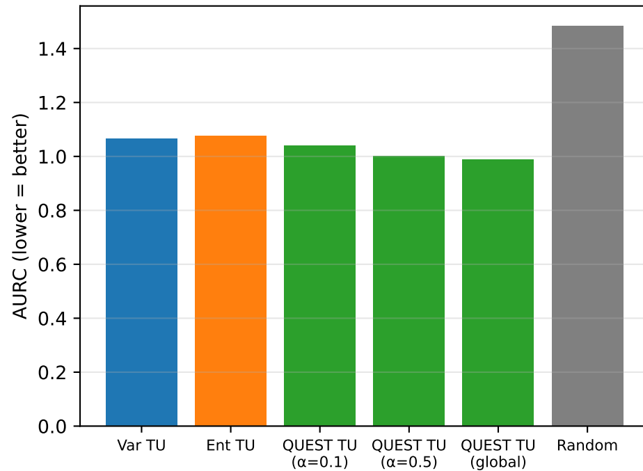
Noise: t5
