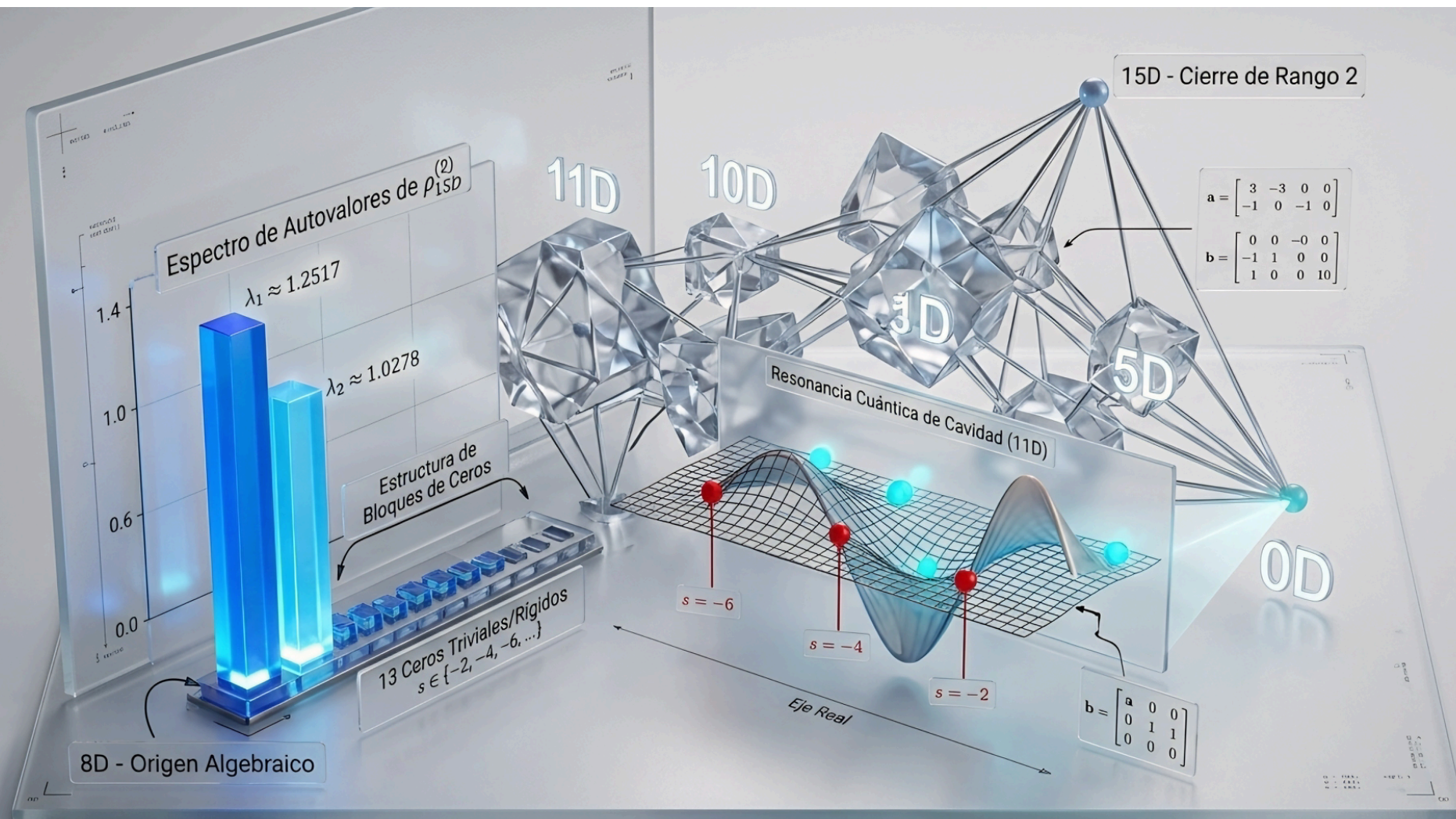
Visualización de la Relatividad Algebraica de Marcos (0D-15D)
