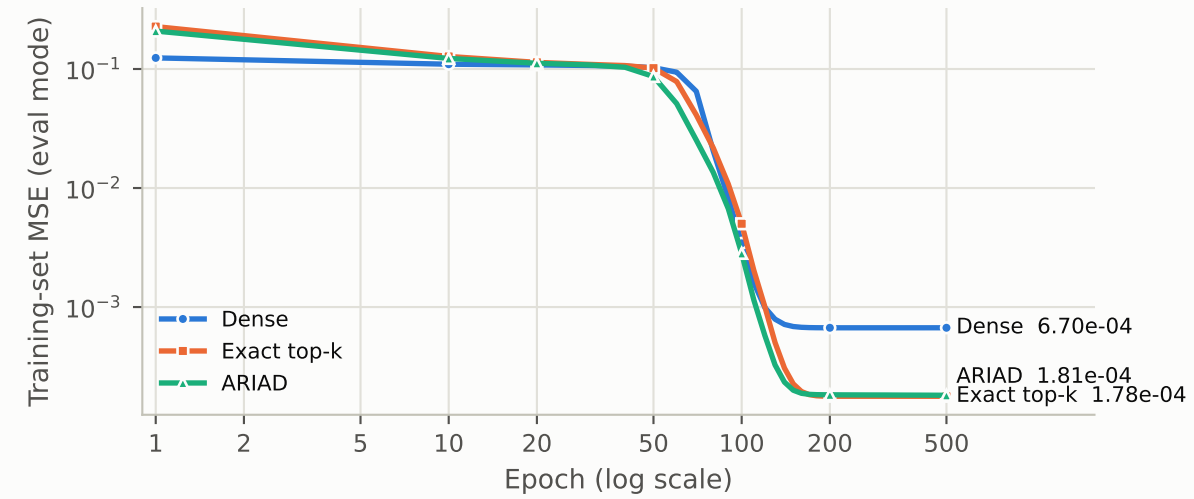
(b) MSE convergence
