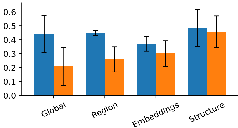
A. Spearman
