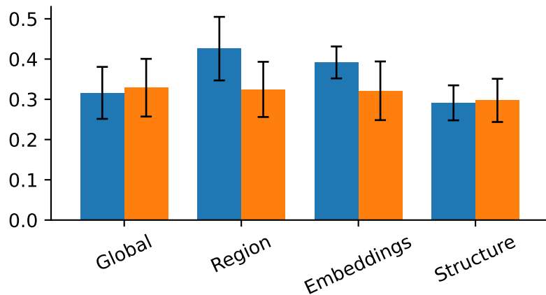
B. RMSE
