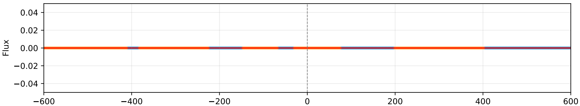
OI 1302
