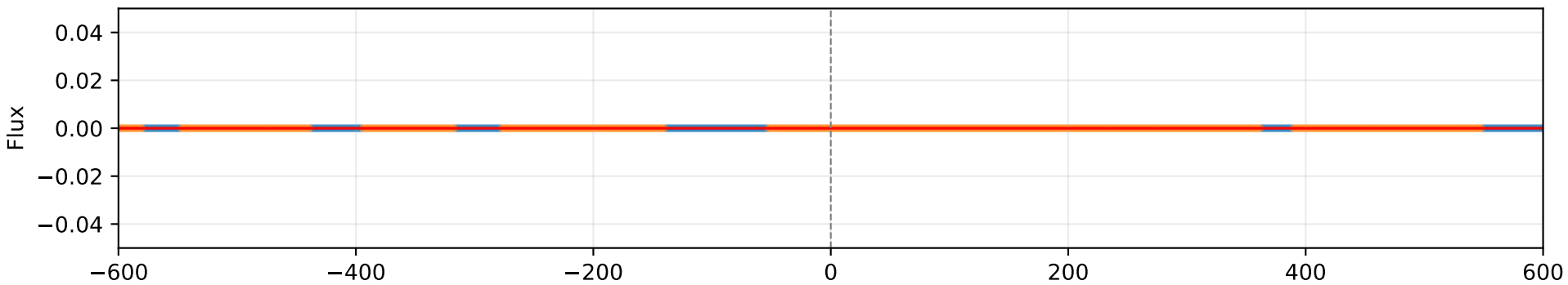
SII 1253
