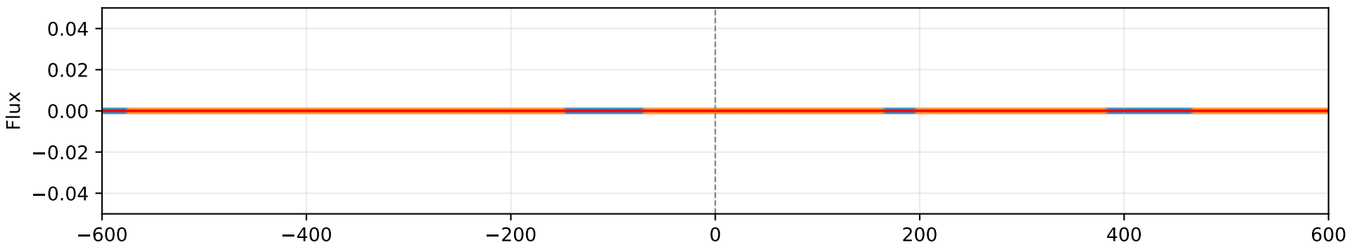
SIII 1526
