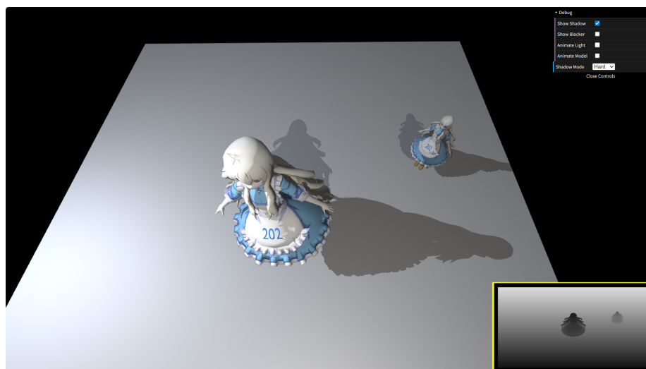
图 1 Shadow Map 硬阴影结果（双光源场景，右下角含 Shadow Map 小窗）
