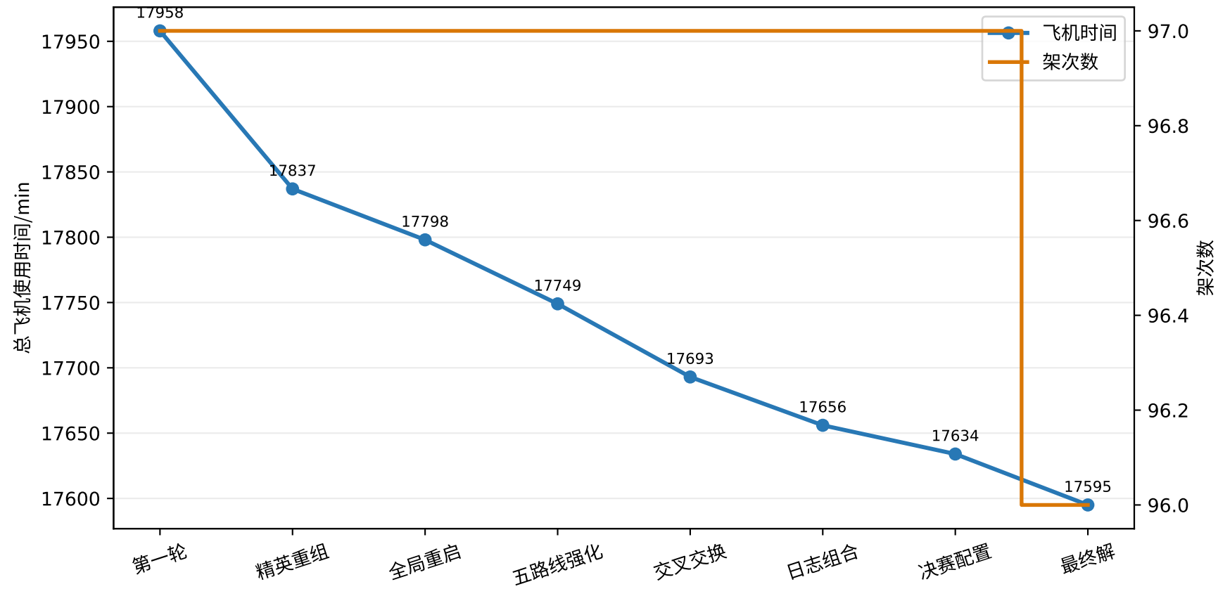
问题二：精确局部重构与多重重启的改进链
