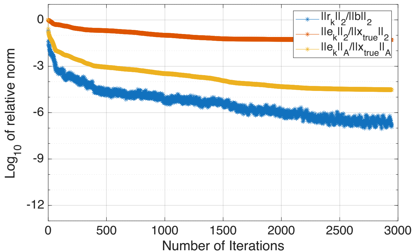
HB/bcsstk12
