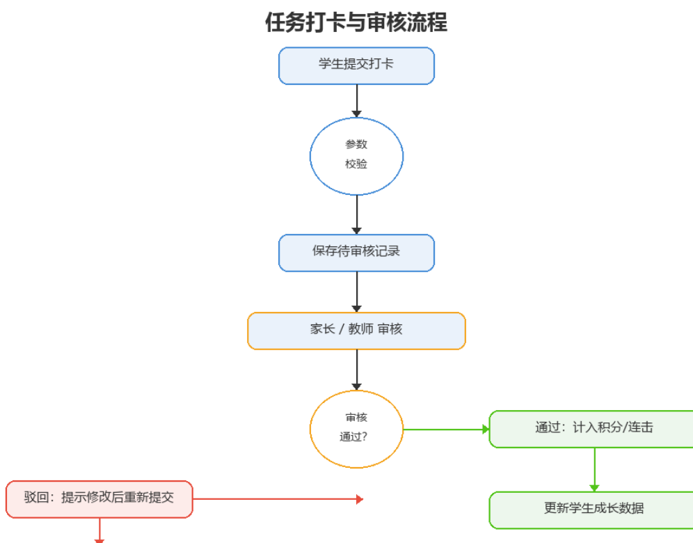
图 7-2 任务打卡与审核流程
