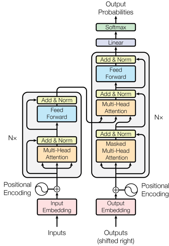
Figura 5.3: Imagen del artículo original donde se muestra la arquitectura del transformador.
