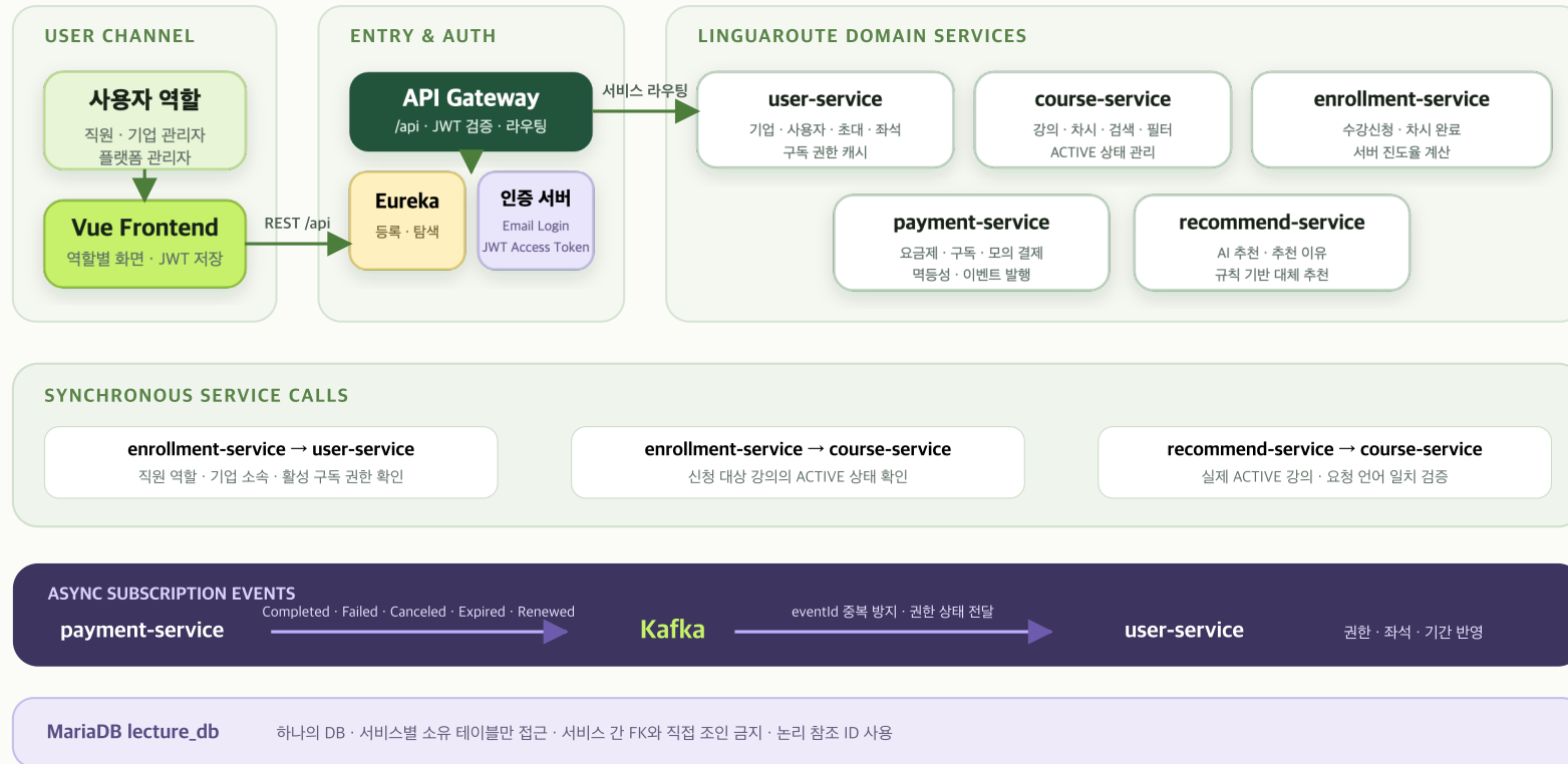
LinguaRoute MSA 아키텍처 구성도
