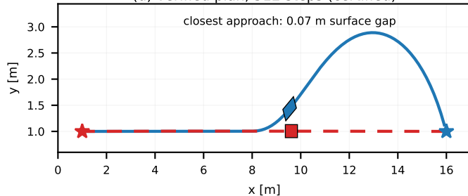
(d) verified plan, 512 steps (certified)
