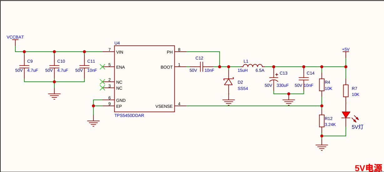
5V电源
