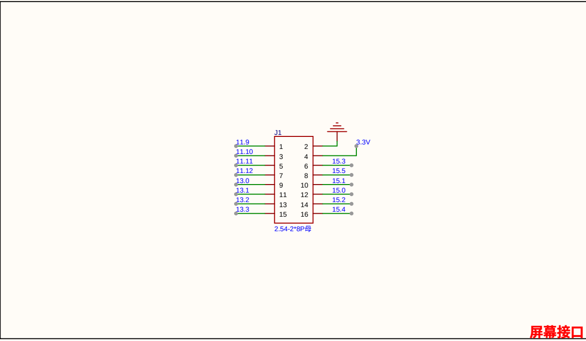
屏幕接口
