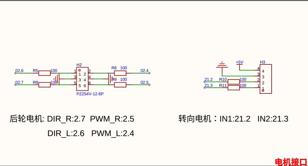
电机接口
