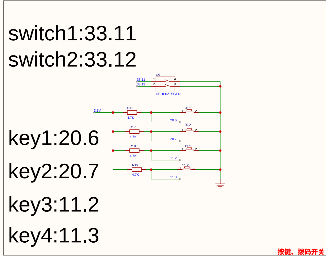
按键、拨码开关
