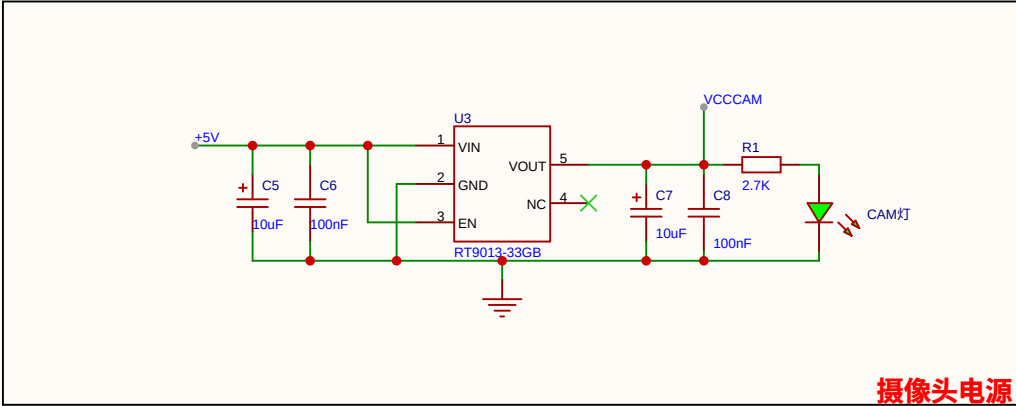
摄像头电源
