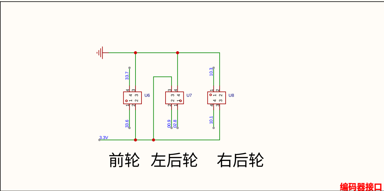
编码器接口
