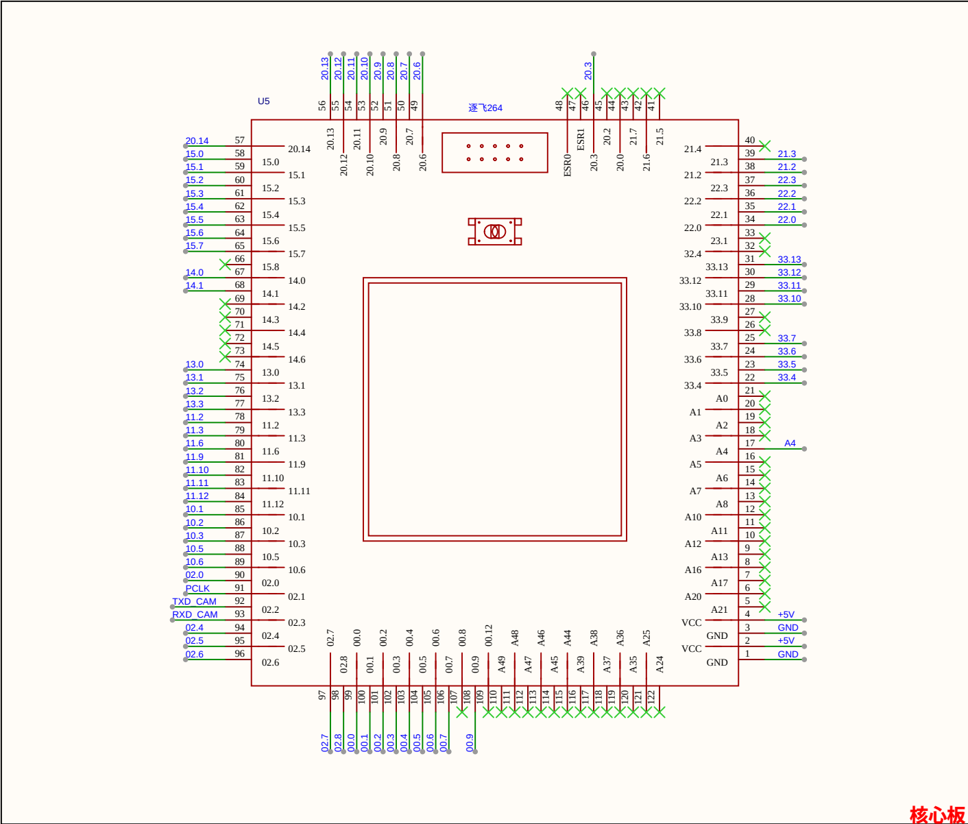
核心板
