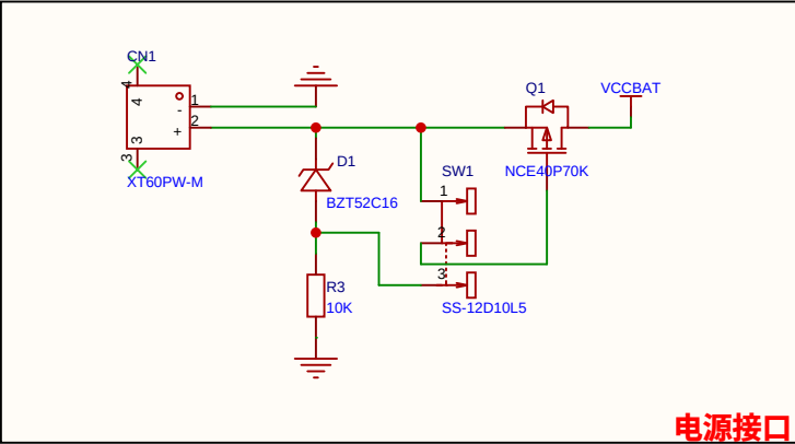
电源接口
