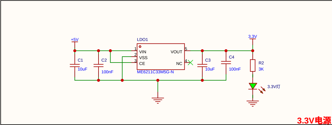
3.3V电源
