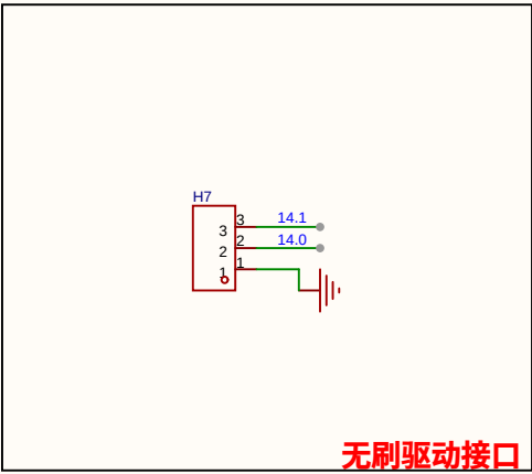
无刷驱动接口
