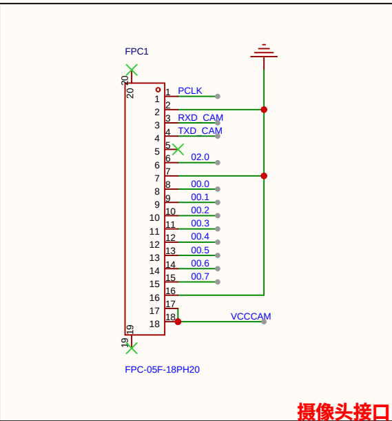
摄像头接口
