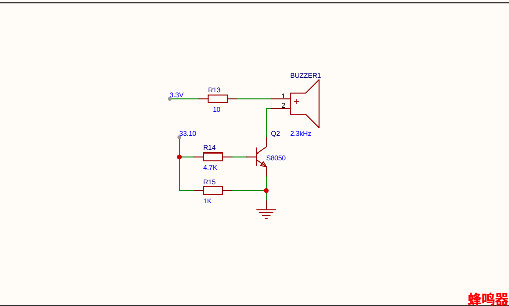
蜂鸣器
