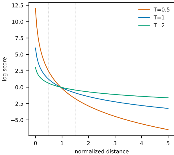
monotone_log
