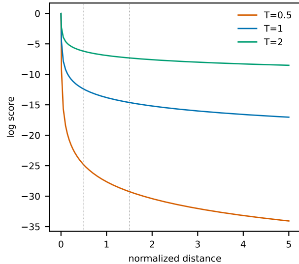
monotone_log
