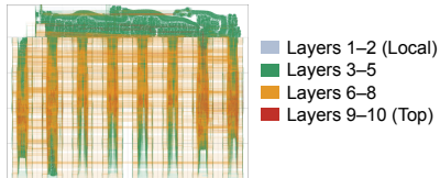
(b) Metal Wiring
