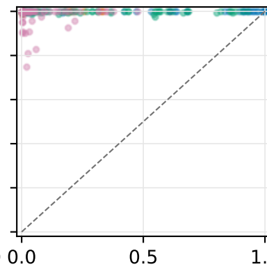
MMLU
