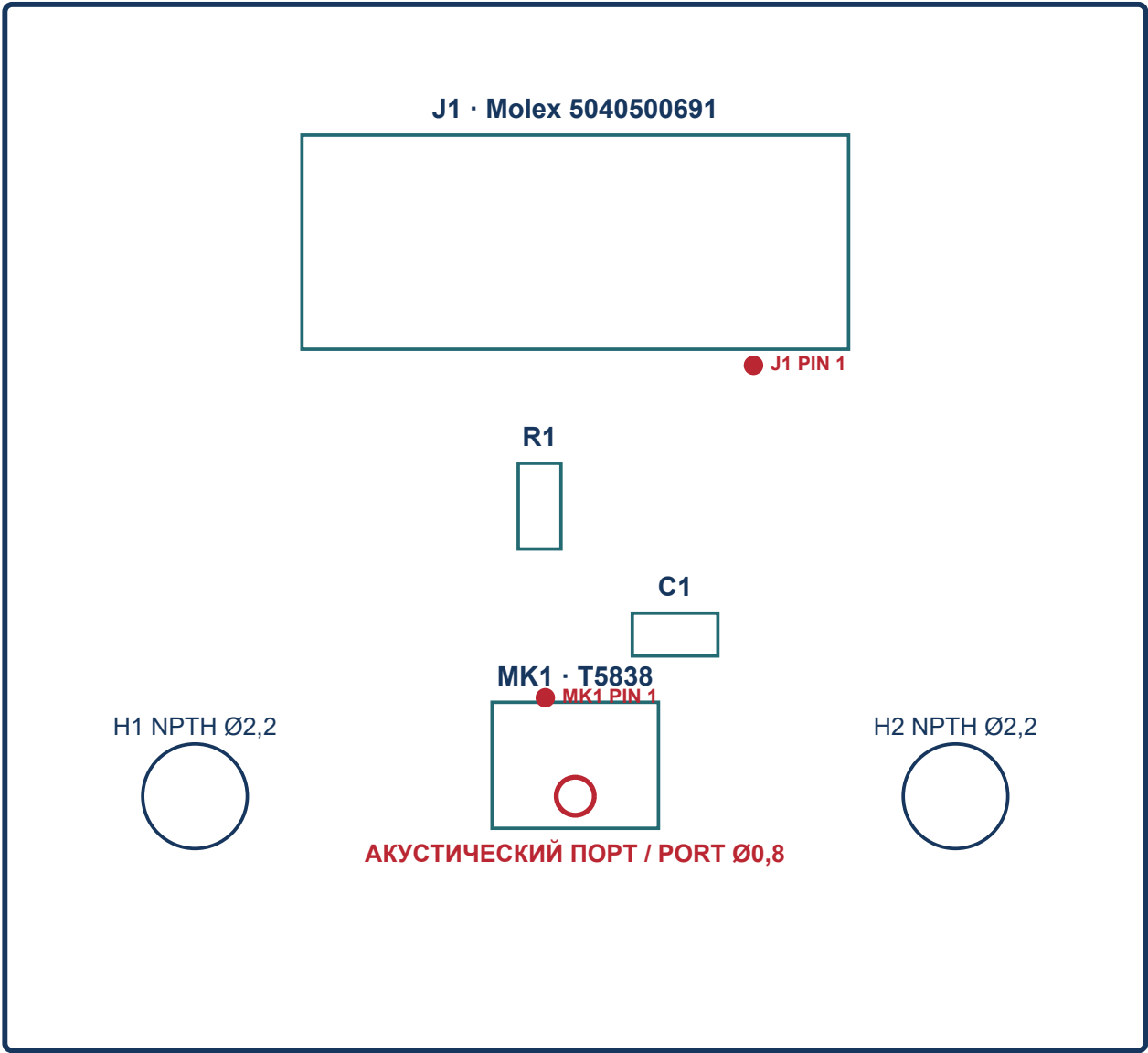
Вид сверху, 19,5 pt/mm / Top view, 19.5 pt/mm; ось Y направлена вниз / Y axis points down Габарит платы / Board outline: 24 × 22 × 1,0 мм; ENIG; 2 слоя / layers
