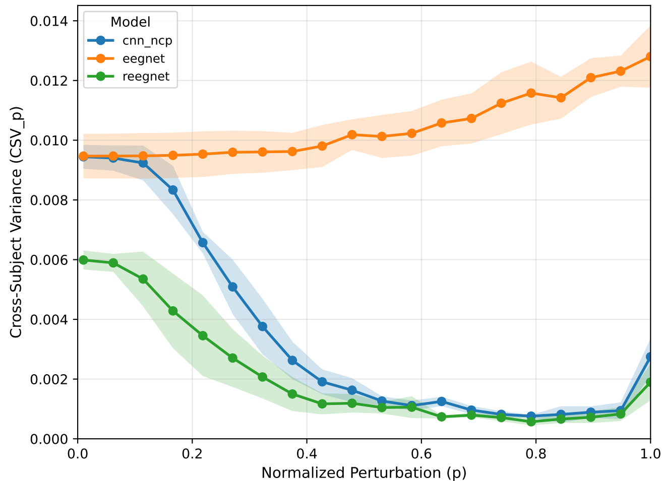
Baseline
