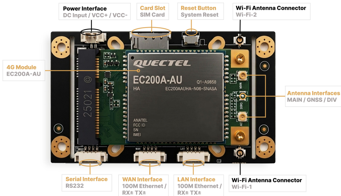
图 3. 正面接口与主要器件布局
