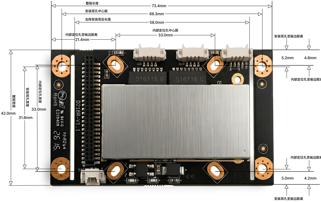
图 6. 产品背面机械尺寸与安装参考
