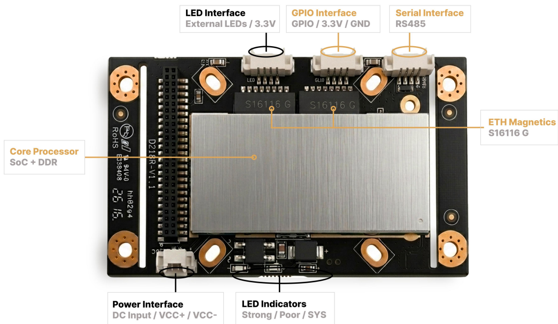
图 4. 背面接口与主要功能区域布局
