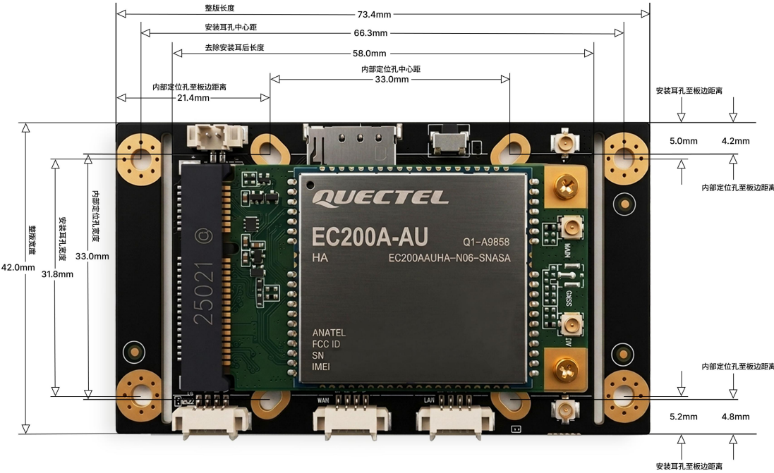
图 5. 产品正面机械尺寸与安装参考
