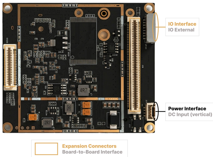
图 4. 背面接口与主要功能区域布局
