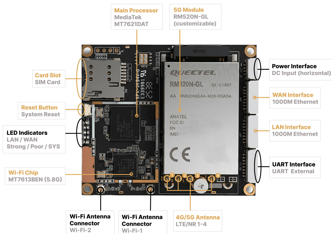
图 3. 正面接口与主要器件布局
