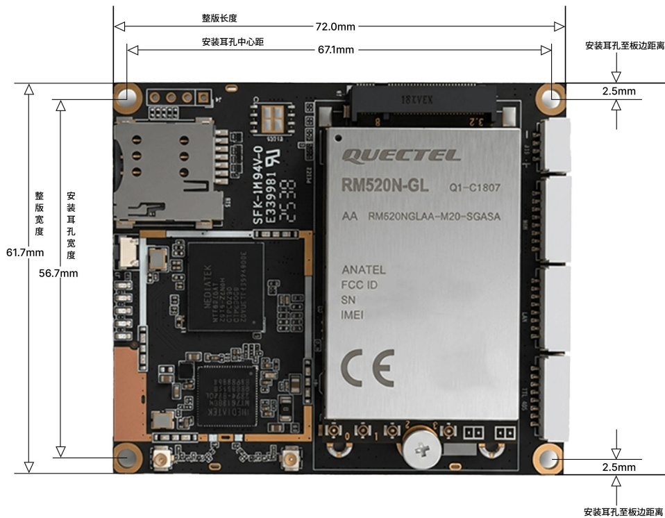
图 5. 产品正面机械尺寸与安装参考
