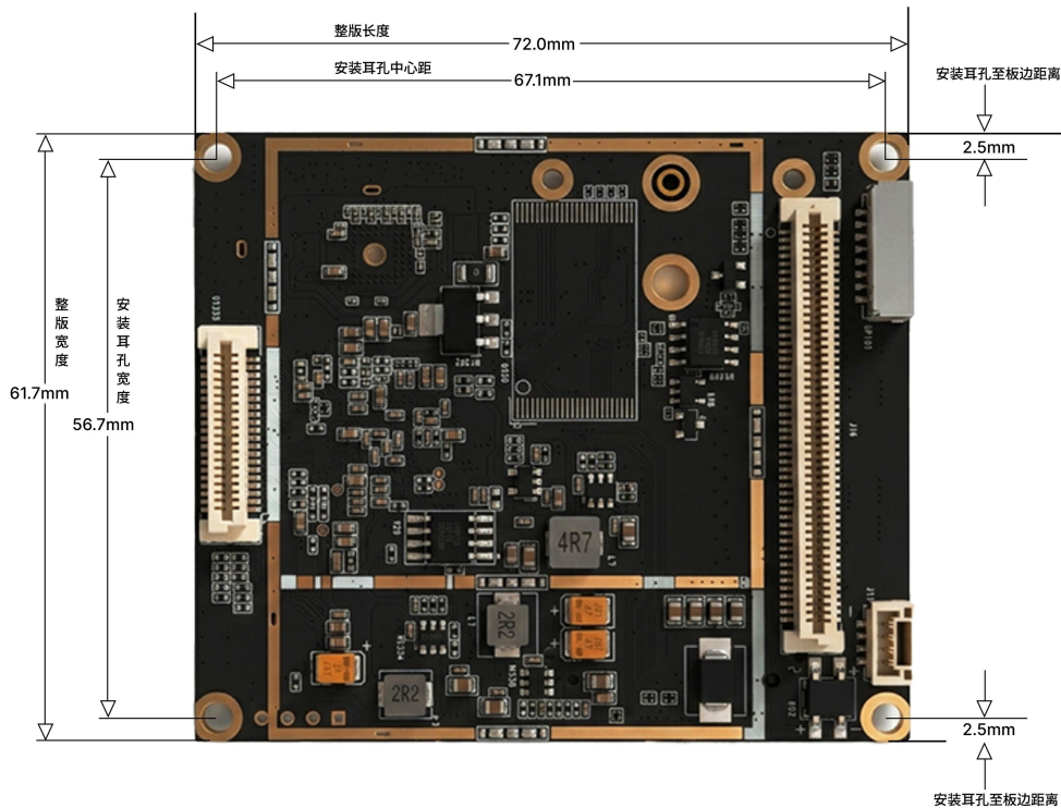
图 6. 产品背面机械尺寸与安装参考
