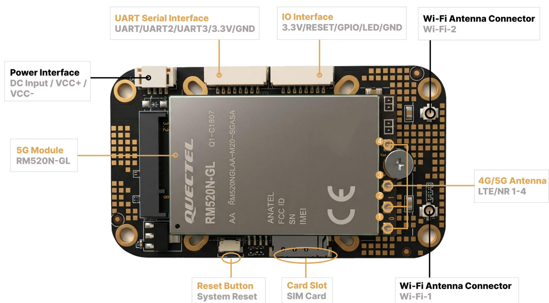
图 3. 正面接口与主要器件布局
