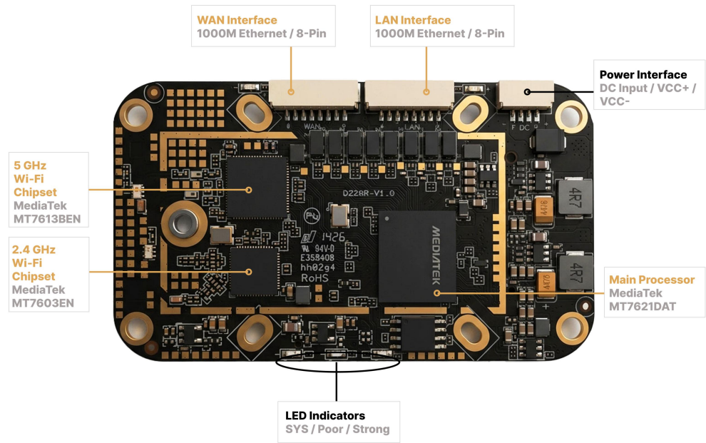
图 4. 背面接口与主要功能区域布局
