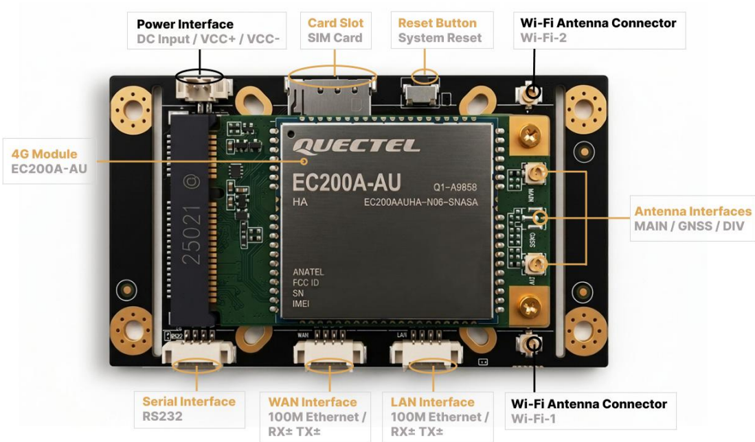
图 3. 正面接口与主要器件布局
