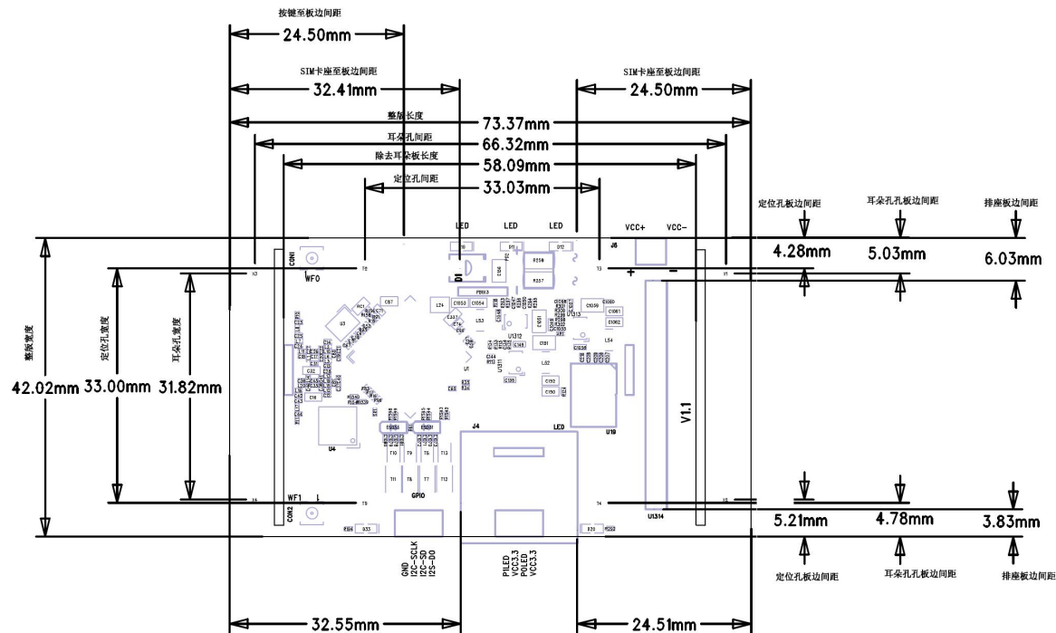
图 5. 机械尺寸图
