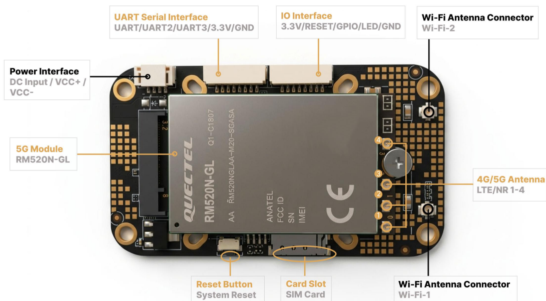
图 3. 正面接口与主要器件布局
