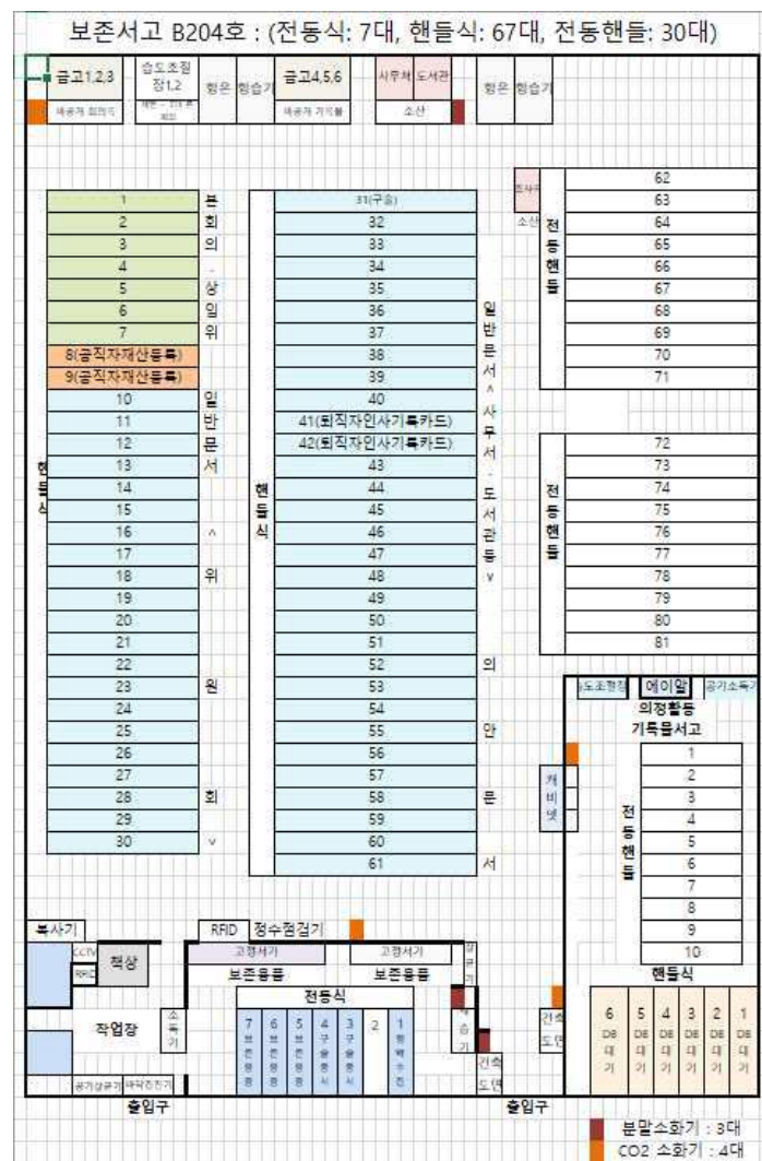
〈그림 33〉 국회기록보존소 보존서고 배치도
