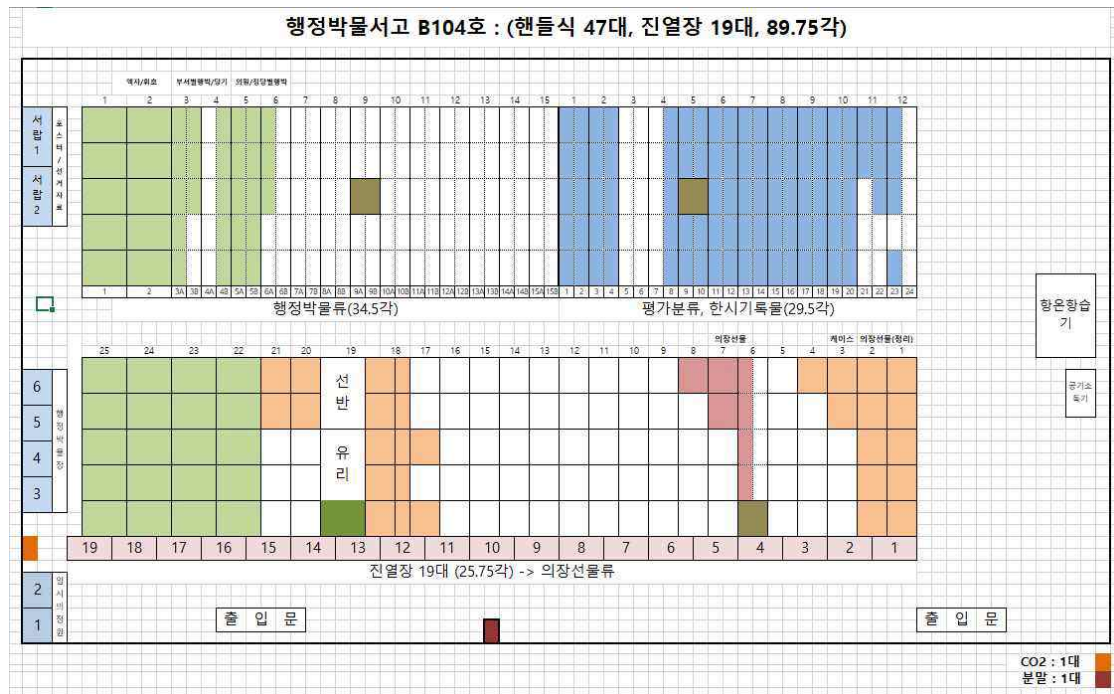
〈그림 34〉 국회기록보존소 행정박물(선물류), 한시기록물 서고 배치도
