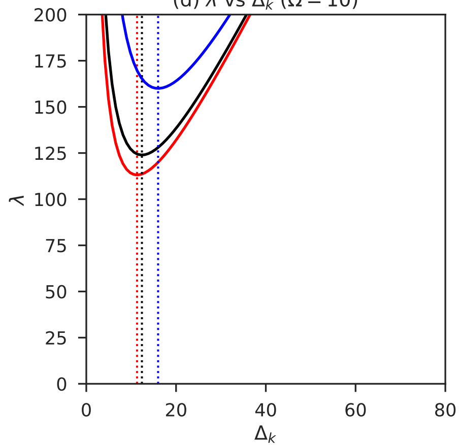
(d) \lambda vs \Delta_k ( \Omega = 10 )
