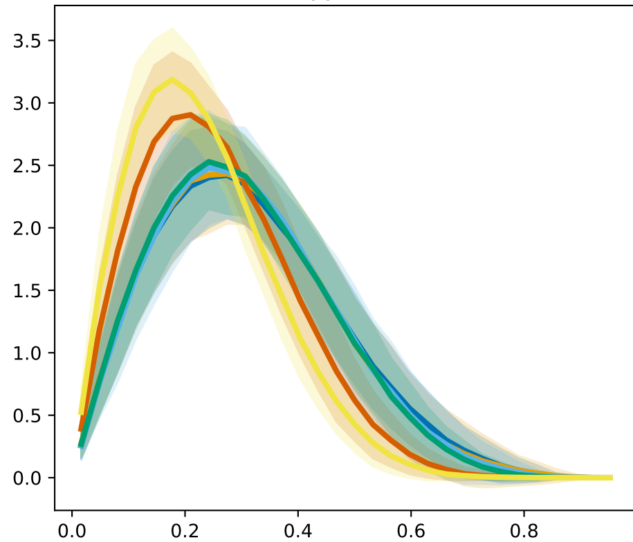
M_A = 2
