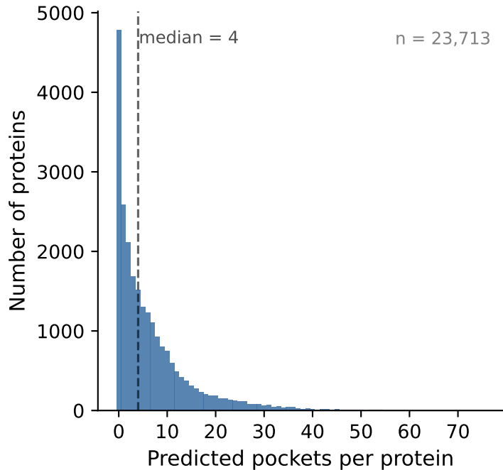
P2Rank
