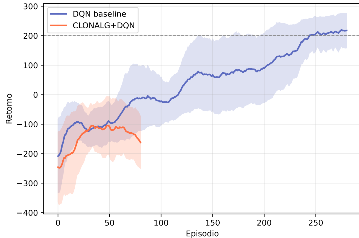
Retorno medio suavizado
