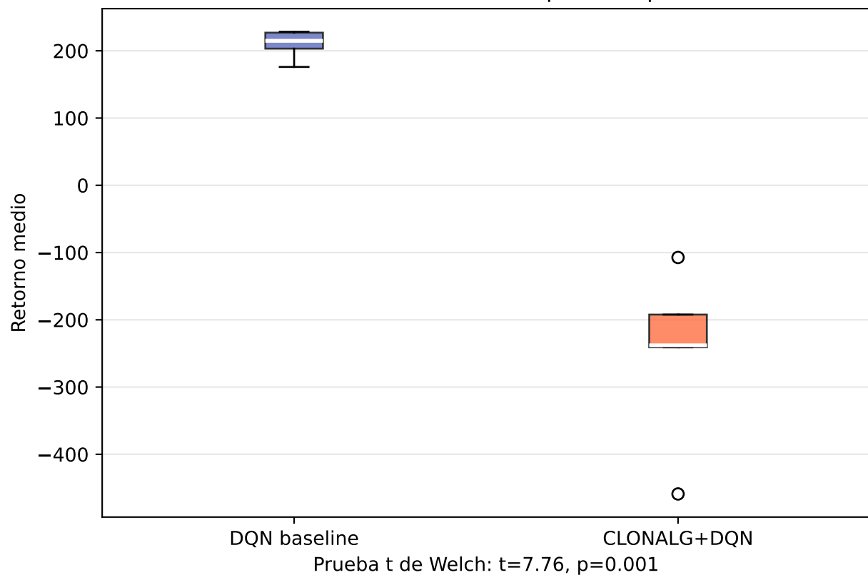
Retorno medio — últimos 50 episodios por semilla
