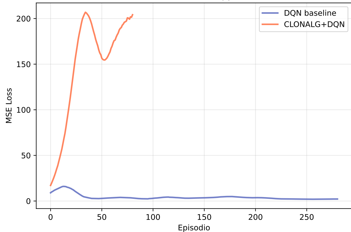
Loss de entrenamiento (clippeada a 500)
