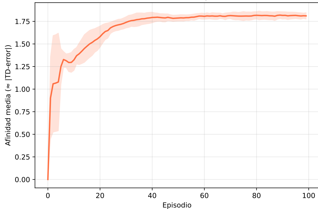
Afinidad media del repertorio
