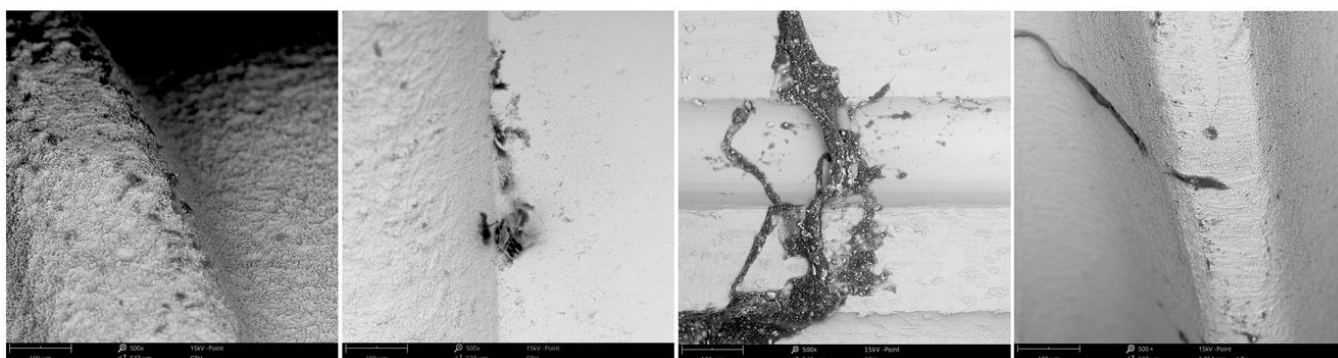
REM-Aufnahmen mit signifikanten Mengen organischer (kunststoffhaltiger) Partikel auf neuen, steril verpackten Zahnimplantaten
