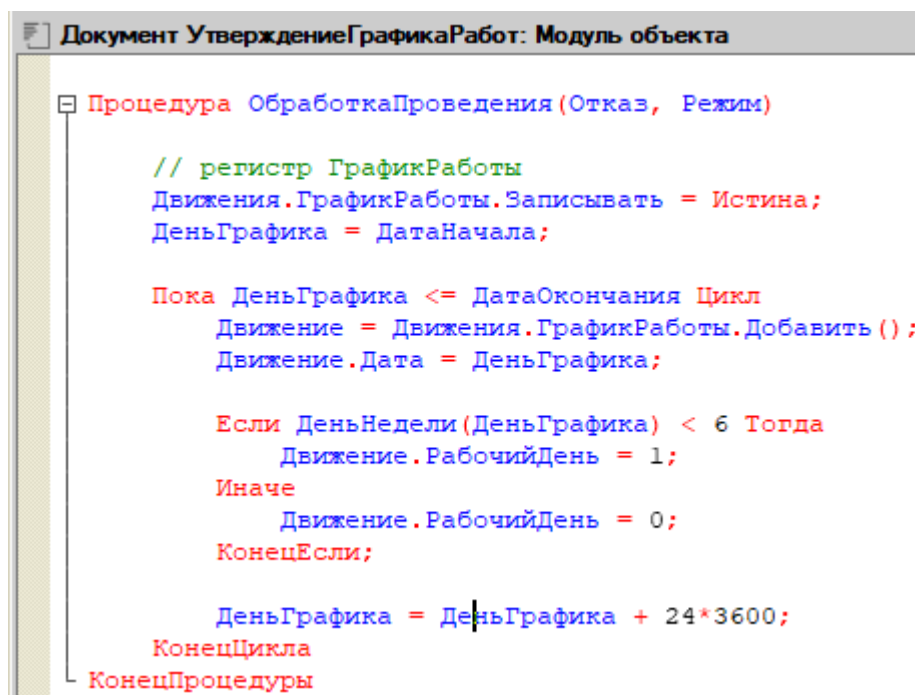
Рисунок 1 – Документ Утверждение графика работ
