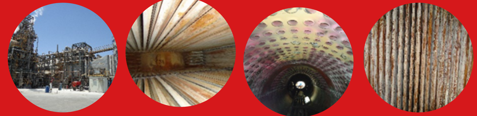
Технологический центр Академии наук Туркменистана – определение технического состояния котла для сжигания отходов.
