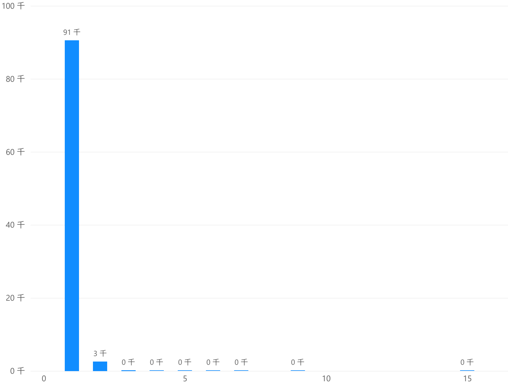
下单次数分布
