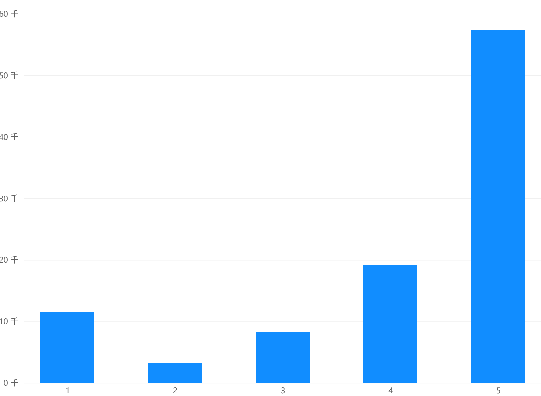
评价分分布（1~5 星） review_score 的计数(按 review_score)
