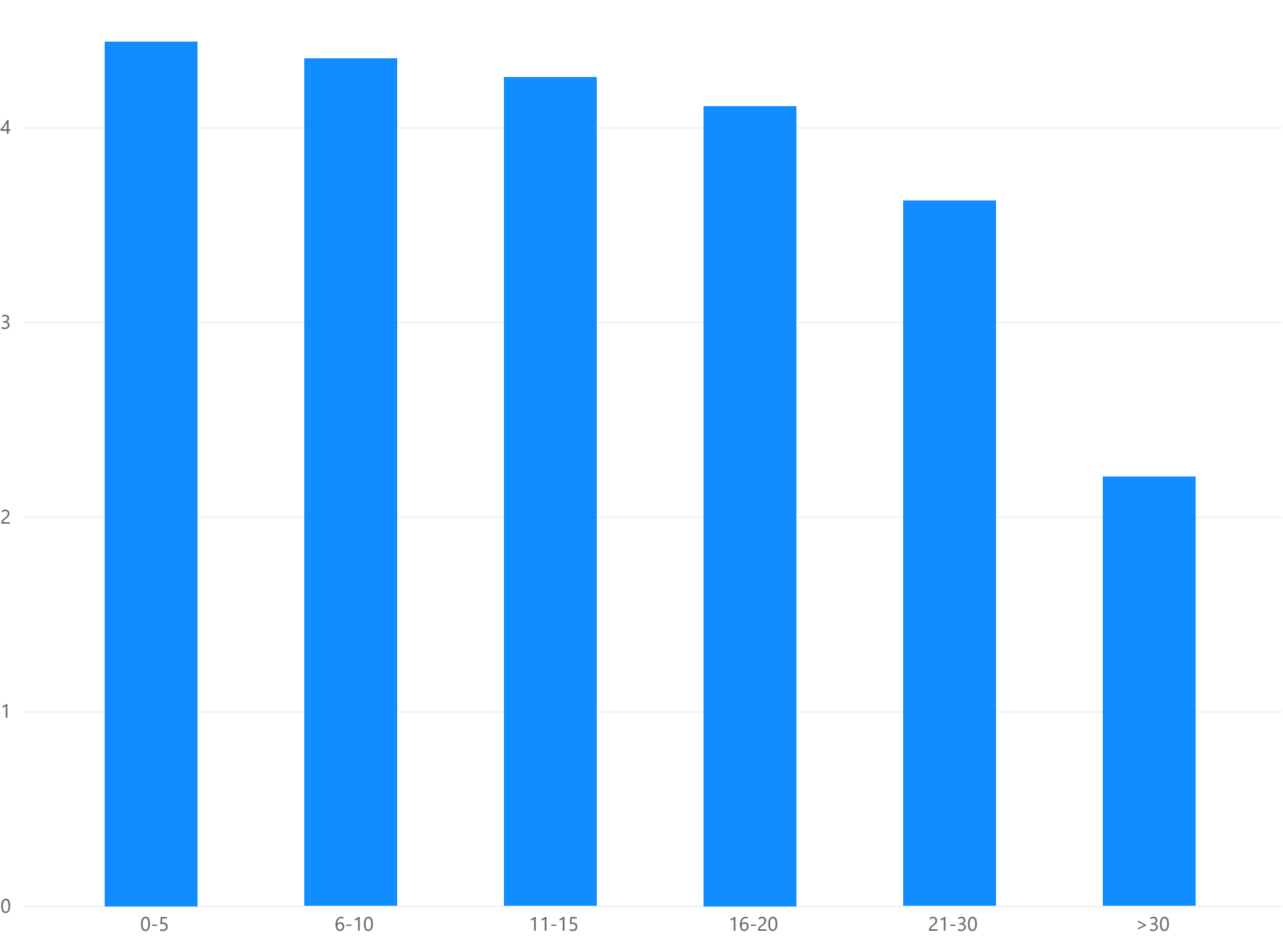
各配送天数分桶的平均评分 Avg Review Score(按 deli_bucket)
