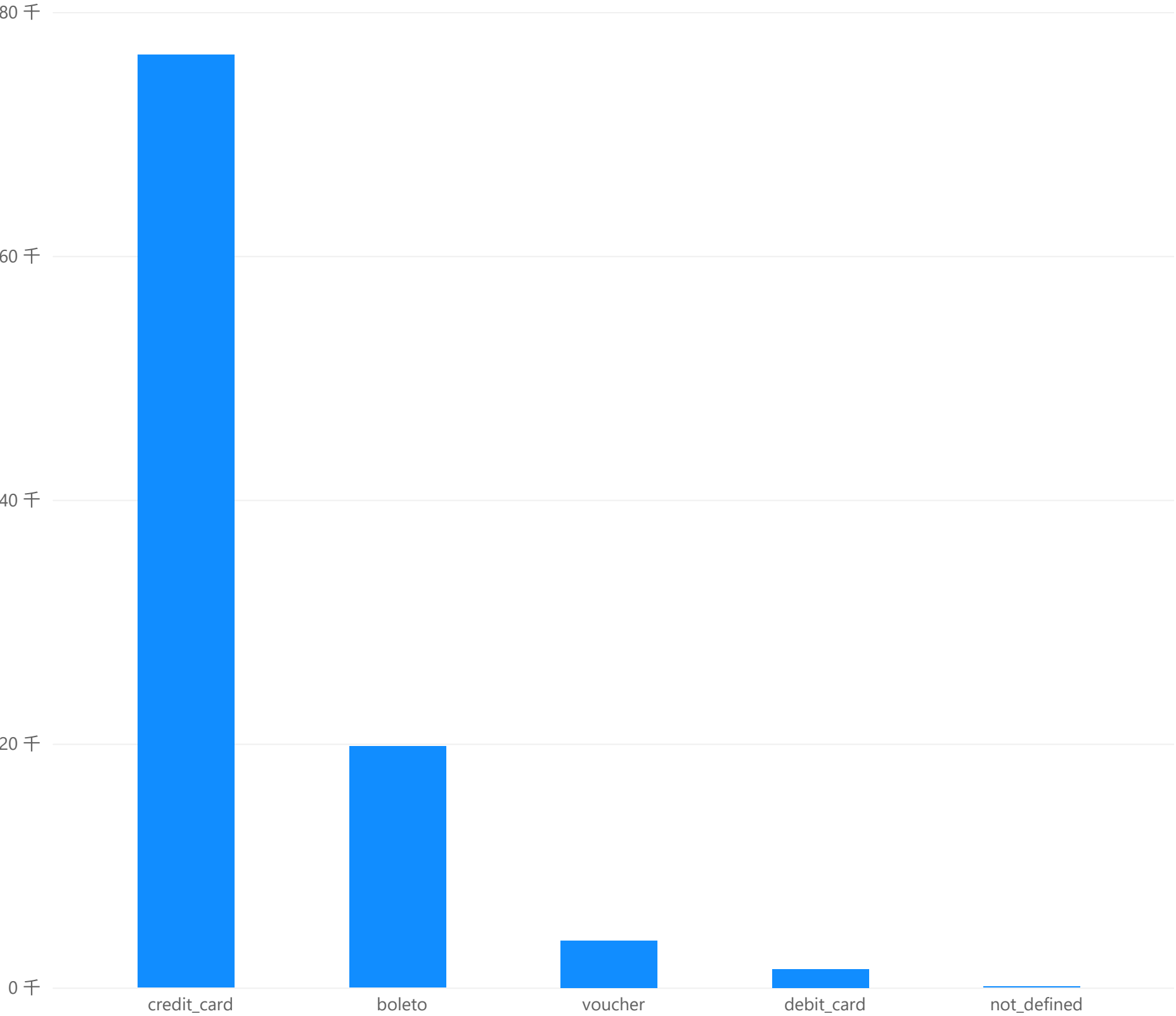
各方式订单数 Payment Orders(按 payment_type)
