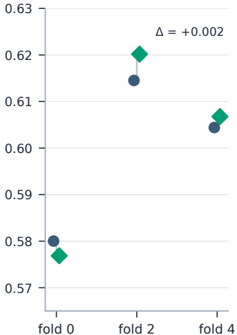
AUPR
