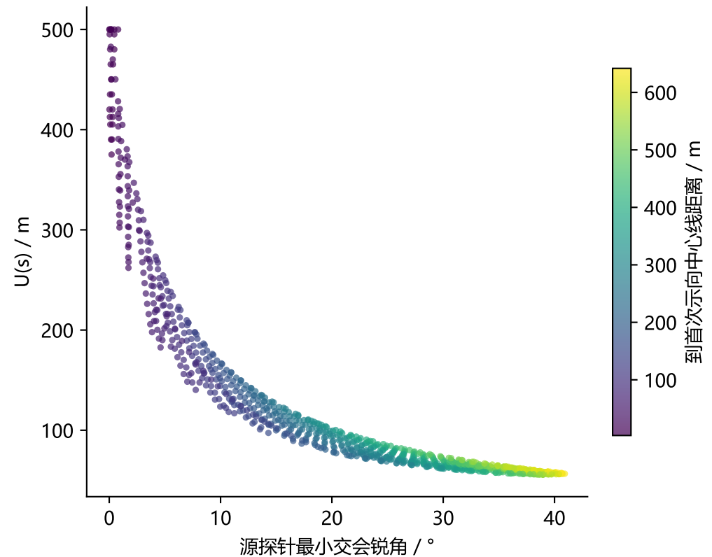
近乎平行的交会放大误差
