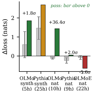
\Delta\text{loss (nats)} ( \uparrow damage)
