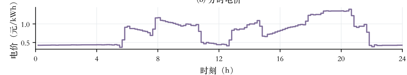
(b) 分时电价
