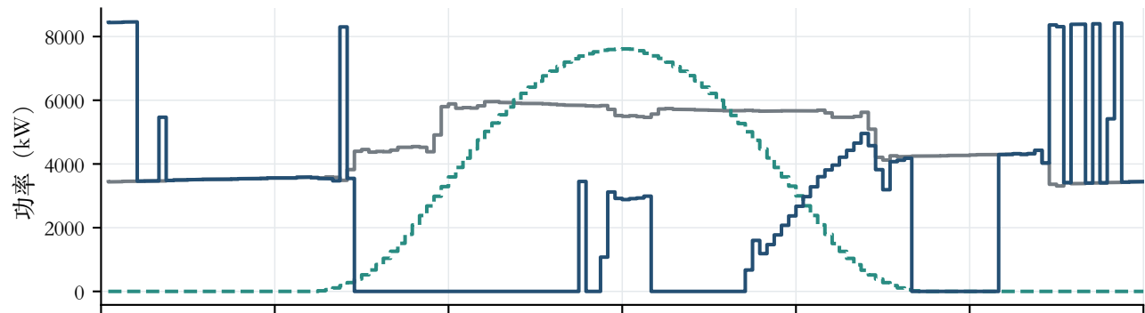
(a) 负载、光伏与购电
