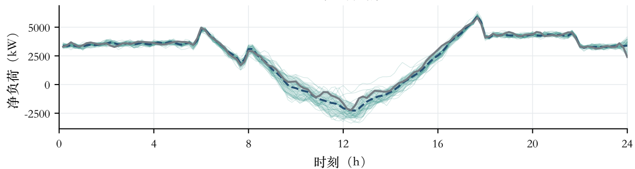
(c) 净负荷场景
