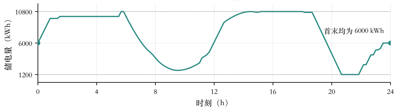
(b) 库存与边界
