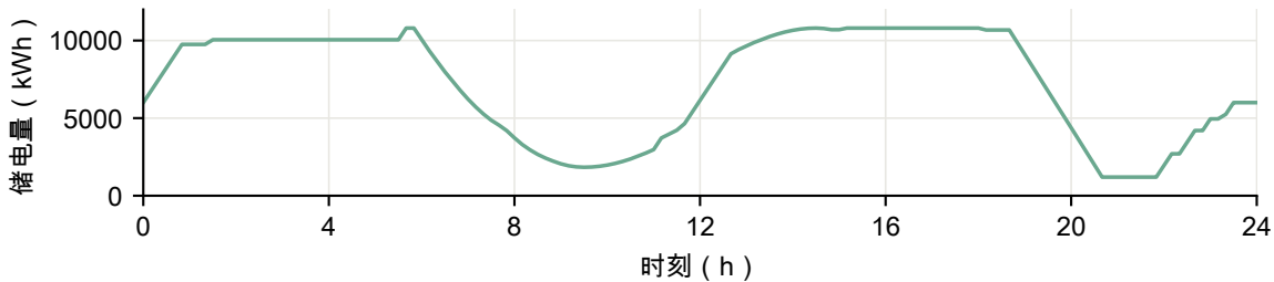
(b) 储电量轨迹
