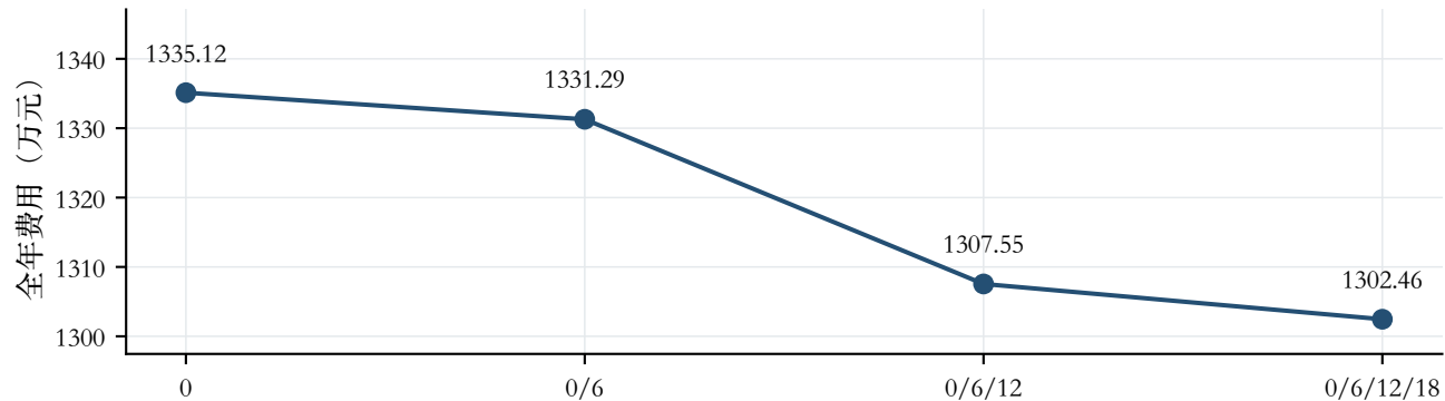
(a) 预报时刻组合 (24h 基线)
