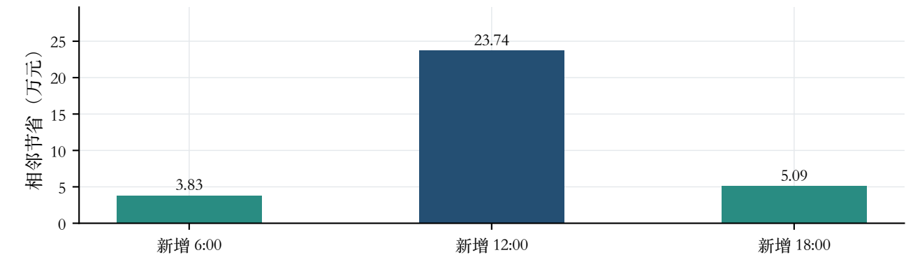
(b) 按固定顺序增加时刻的节省
