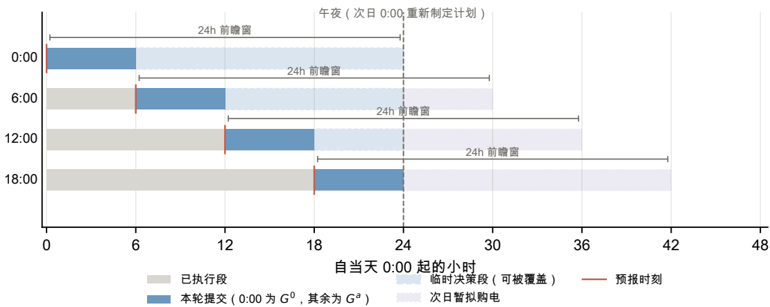
图 8 滚动重优化时间线：四个发布时刻各前瞻完整 24 小时（可跨午夜），实际只提交到下一发布时刻（实色段），其后为可被覆盖的临时决策（虚框段）
