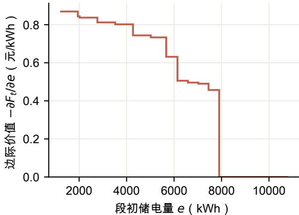
(b) t = 12:00 的边际价值 ( 非增阶梯 )
